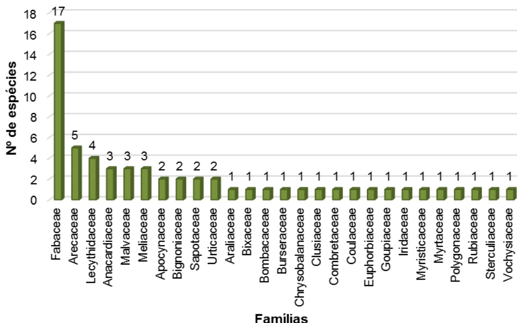
Gráfico 1 – Número de espécies por família
